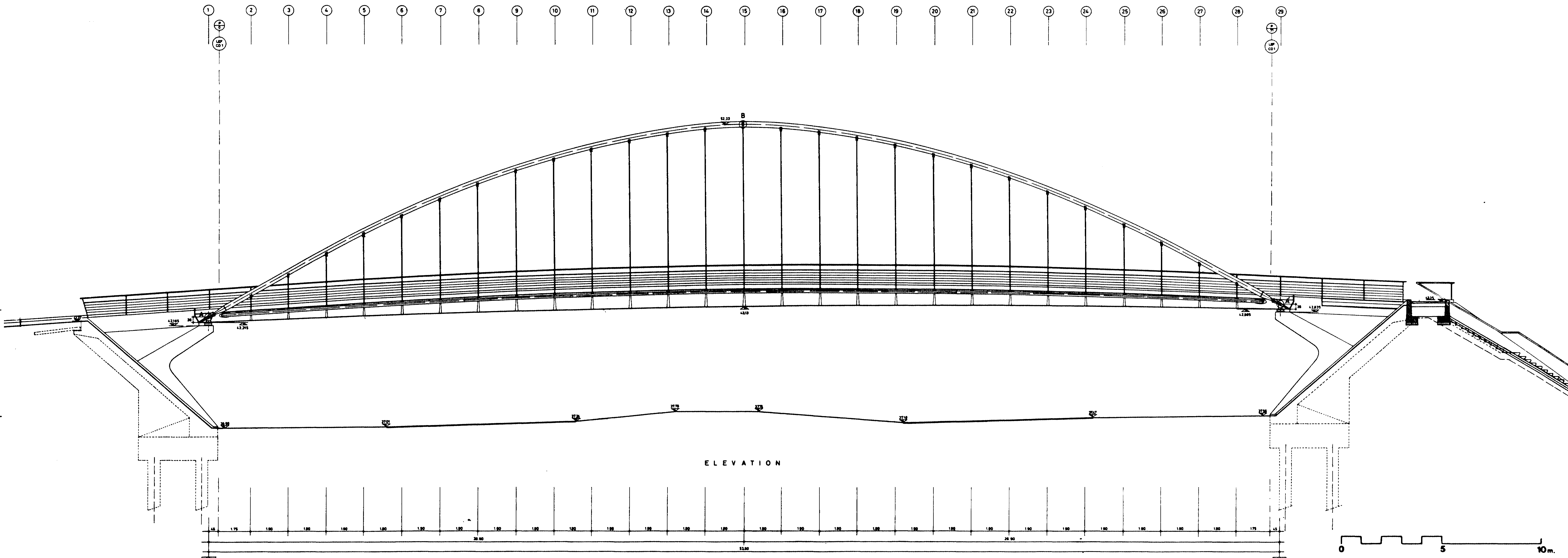
Alzado / Elevation
