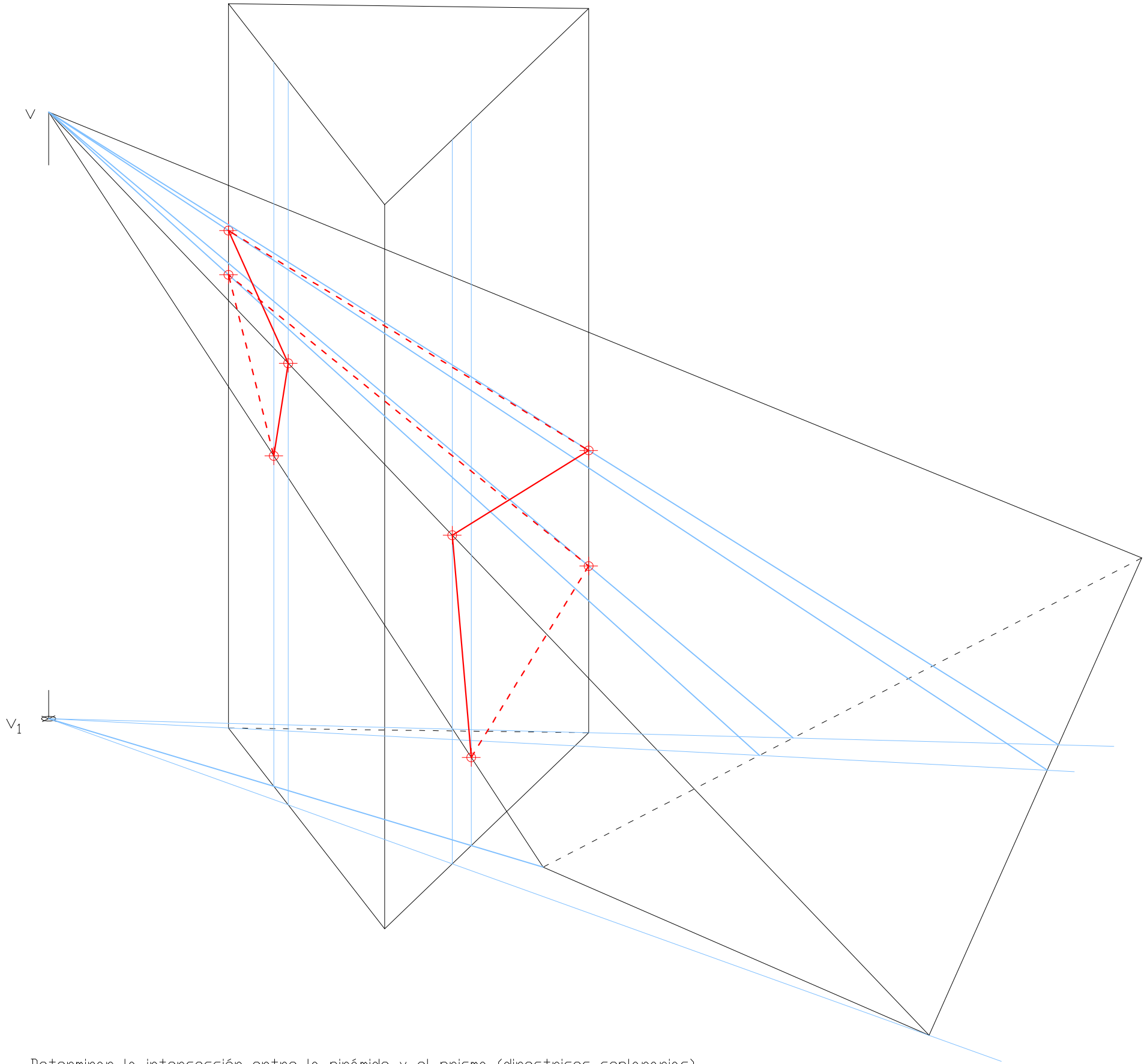
Determinar la intersección entre la pirámide y el prisma (directrices coplanarias)
